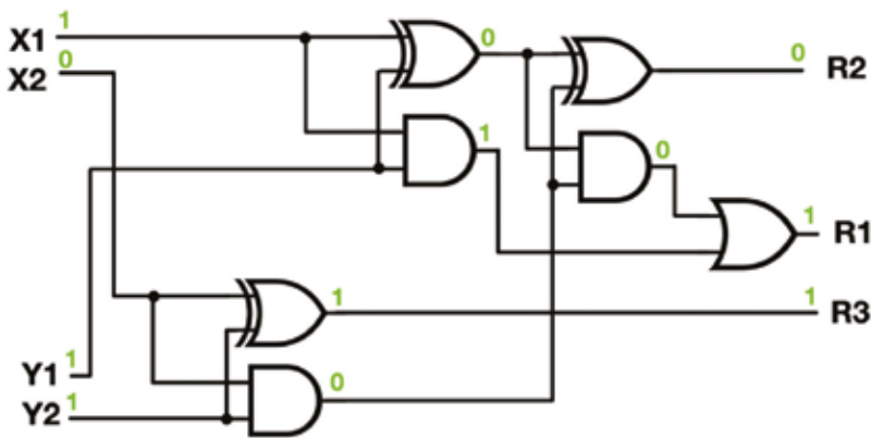
FIGURA 8. DIAGRAMA de circuito de una computadora que permite sumar dos números del conjunto (0,1,2,3) en binario: X1X2 + Y1Y2 = R1R2R3 . Por ejemplo, (2+3)_{\text{decimal}} = (10+11)_{\text{binario}} = 101_{\text{binario}} = 5_{\text{decimal}} .
