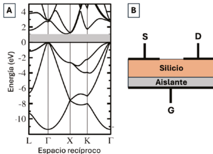
FIGURA 3. ESTRUCTURA de banda del silicio (Fuente: physics.stackexchange.com) y diagrama de construcción de un transistor de efecto de campo basado en silicio.
