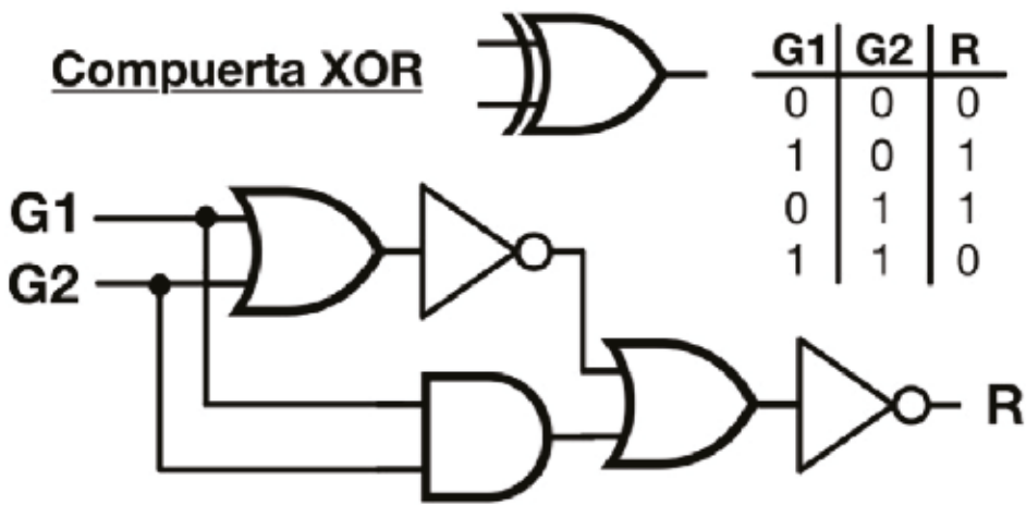
FIGURA 5. USANDO las compuertas mostradas en la Figura 4, podemos construir más compuertas lógicas, como la compuerta XOR.
