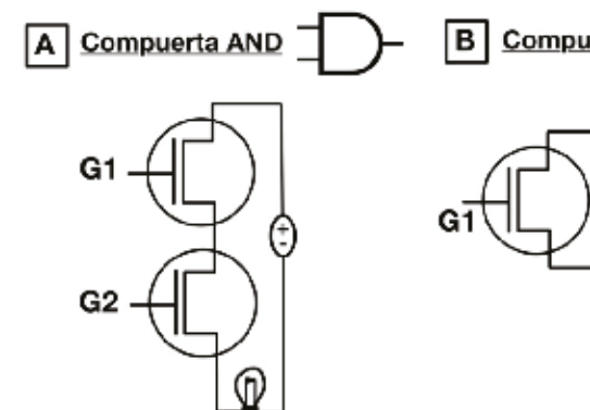
Analizamos ahora el siguiente circuito FIGURA 4. LOS circuitos de transistores permiten realizar operaciones de la lógica. Se muestran las compuertas AND, OR y NOT.
