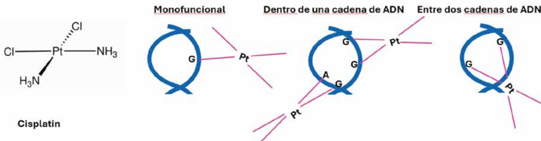
FIGURA 1. LA estructura de Cisplatino y su interacción con cadenas de ADN. Izquierda, la estructura del Cisplatino (tomada de https://en.wikipedia.org/wiki/Cisplatin ). Restantes figuras, tres maneras de interacción del cisplatino con las cadenas de ADN (en azul). G, guanina, A, adenina. Los esquemas de la interacciones se dibujaron con información publicada en (6).
