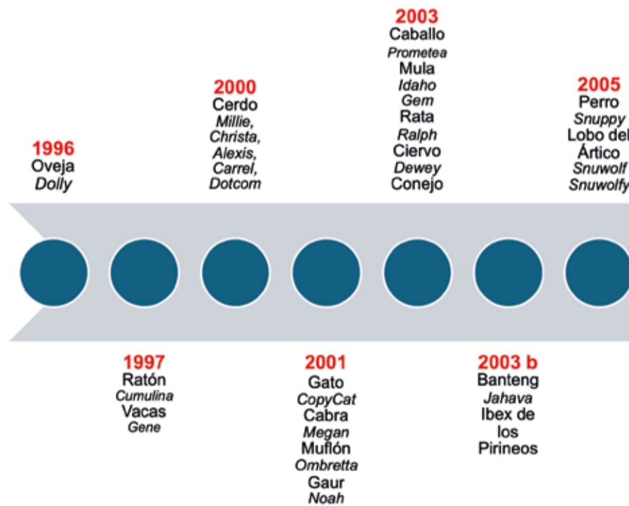
FIGURA 2. APLICACIÓN exitosa de la tecnología de TNCS (o sus variantes) a veintitrés mamíferos. Se muestra en rojo el año de éxito para el animal correspondiente, en cursivas el nombre asignado a las clonas producidas. Elaboración propia con información de https://en.wikipedia.org/wiki/List_of_cloned_animals y referencia (2).
